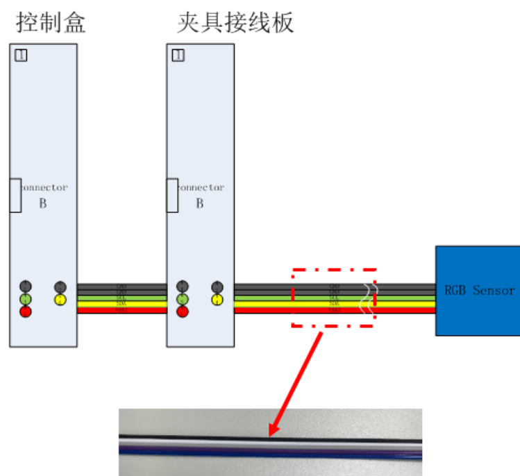
图 4.6 RGB 接线示意图
