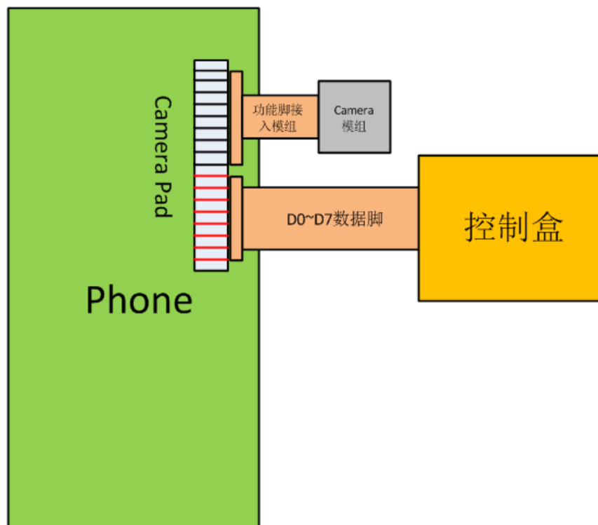
图 4.4 MCU camera 接线示意图
