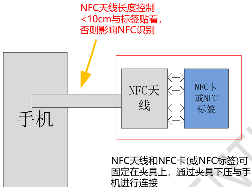
图 4.8 NFC 夹具连接示意图
