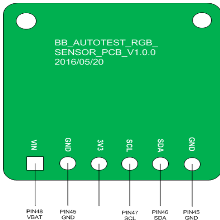
图 4.7 RGB Sensor 结构示意图
